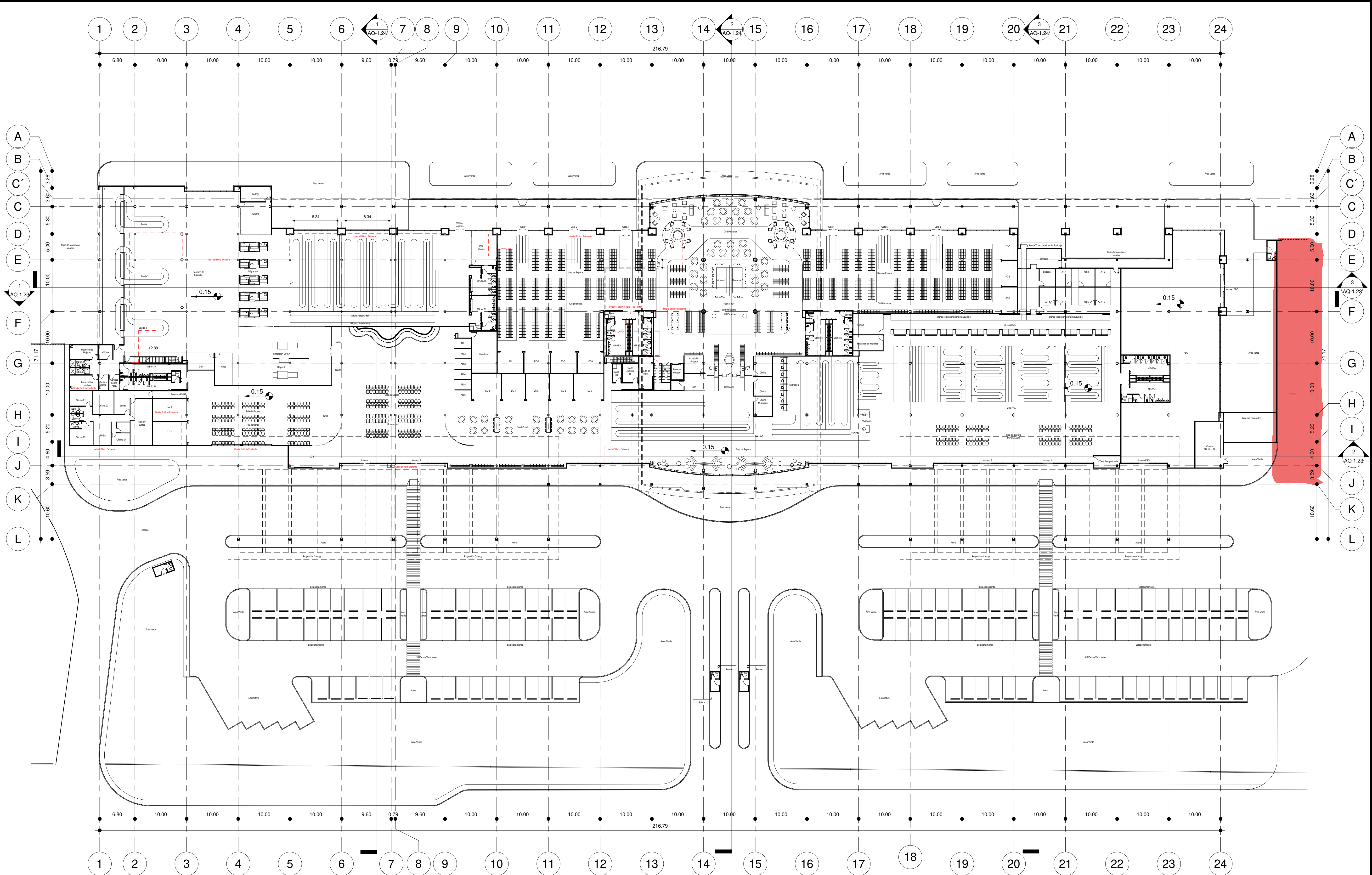
1 Planta Arquitectónica Nivel 1 1 : 350
